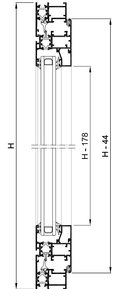
Sección B-B'
